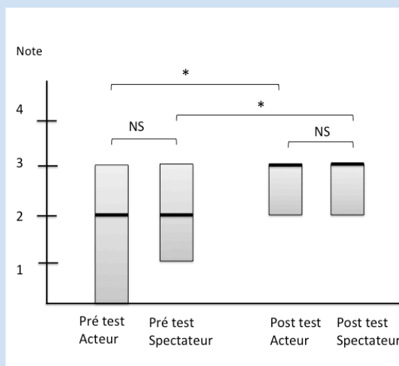
Figure 1 : résultats des tests avant et après la simulation en fonction du rôle d'acteur ou spectateur au scénario évalué. Les résultats ont été exprimés en médiane [espace interquartile].
